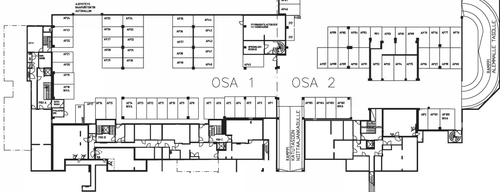
ASA OY MERENIKKUNA KELLARIKERROS K1
